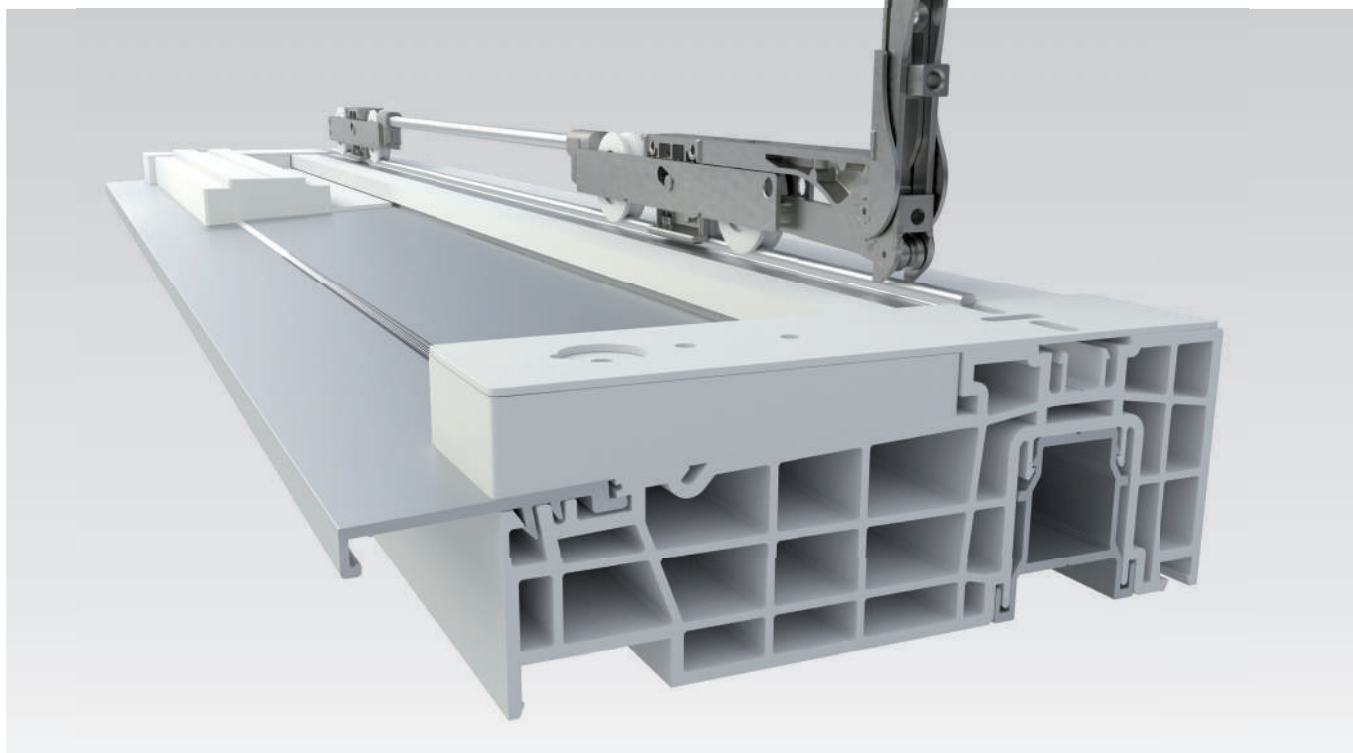
Bodenschwelle auf höchstem Vorfertigungsgrad vormontiert (oben abgebildet GU-thermostep 204 für Holzelemente)
